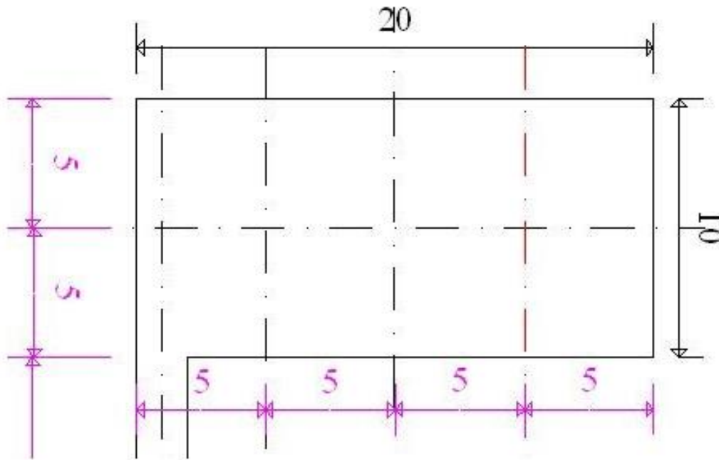
Mesures de la Chambre du Roi
