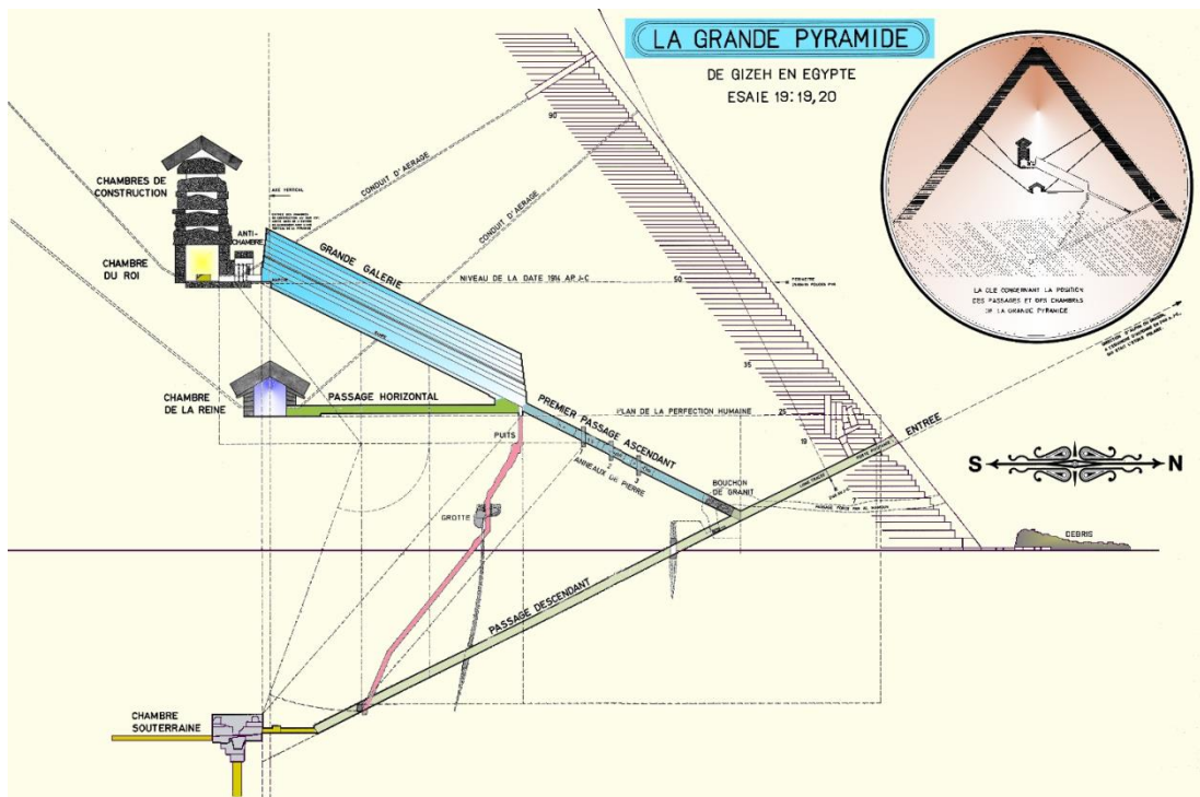
Schéma des Couloirs et des Chambres de la Grande Pyramide
